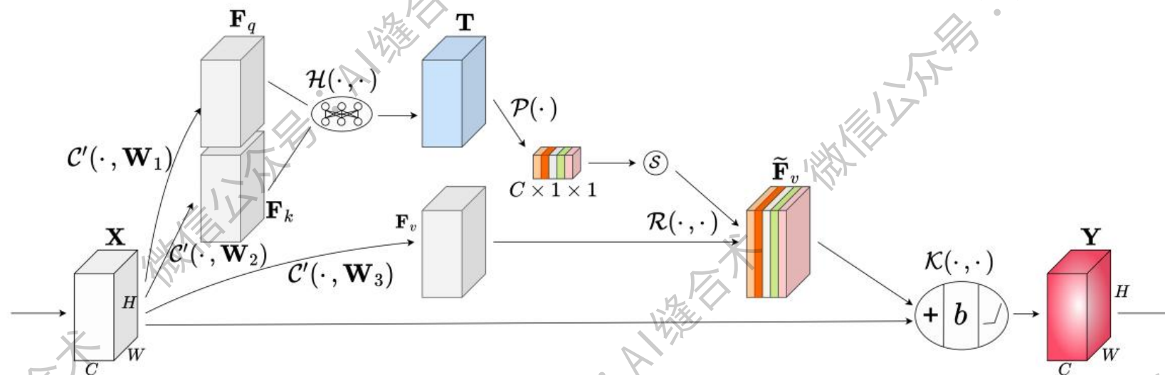
Figure 2. CSA-ConvBlock.
